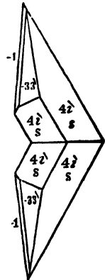
Schwarzenstein.
